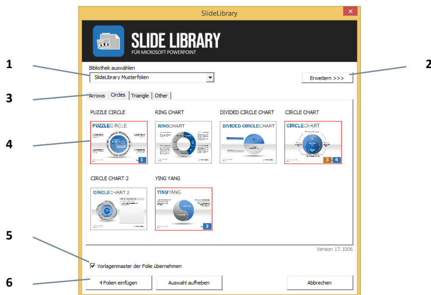
Abbildung 12: SlideLibrary Hauptdialog
